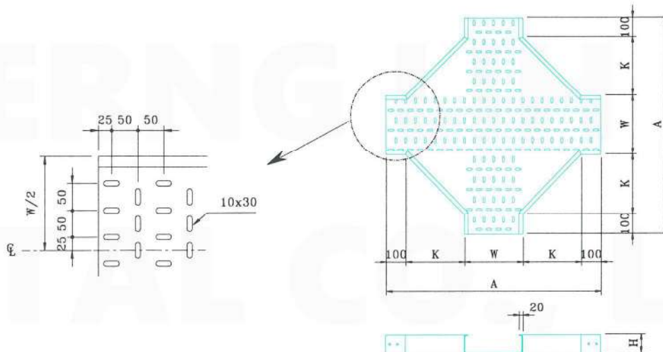
邊槽高度 60H 系列 (60mm HEIGHT SERIES) 厚度 (T)=1.6mm or 2mm
