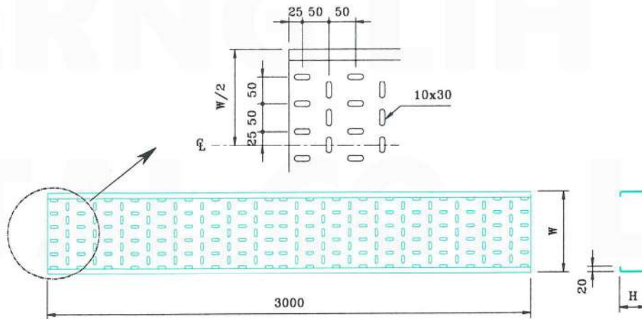
邊槽高度 60H 系列 (60mm HEIGHT SERIES) 厚度(T)=1.6mm or 2mm
