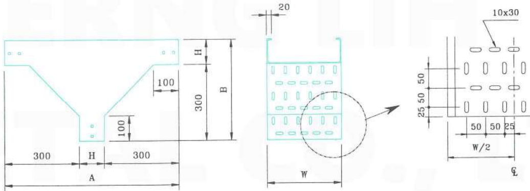
邊槽高度 60H 系列 (60mm HEIGHT SERIES) 厚度 (T)=1.6mm or 2mm
