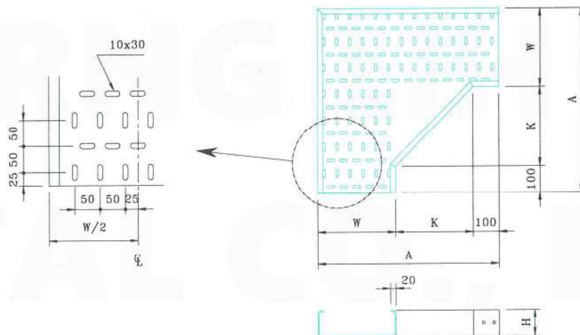
邊槽高度 60H 系列 (60mm HEIGHT SERIES) 厚度 (T)=1.6mm or 2mm
