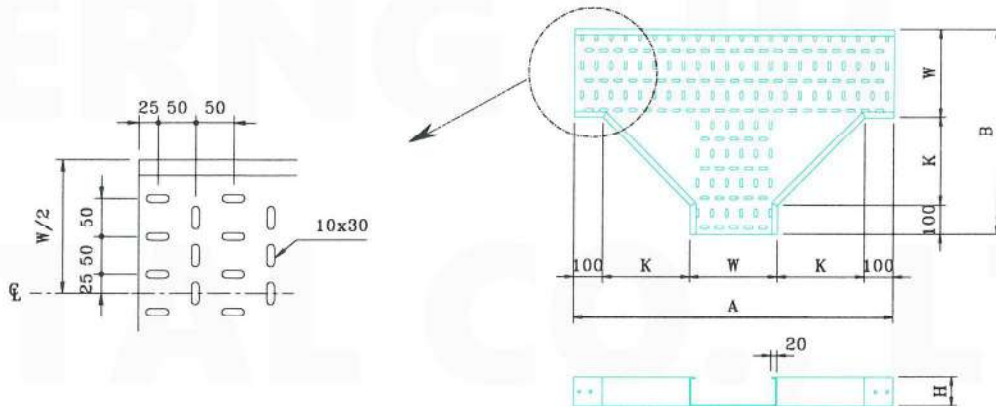
邊槽高度 60H 系列 (60mm HEIGHT SERIES) 厚度 (T)=1.6mm 或 2mm
